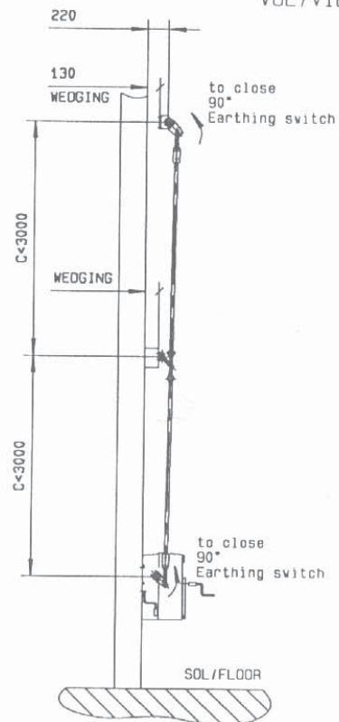
VUE / VIEW A
