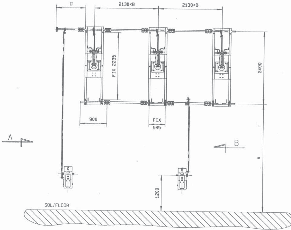
VUE / VIEW A
