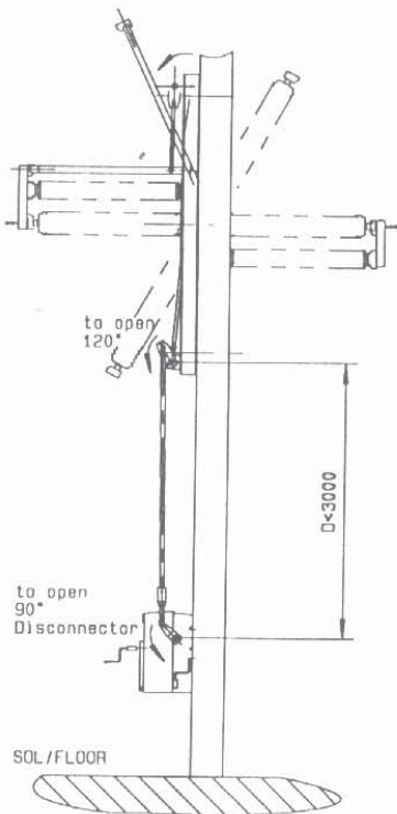
VUE / VIEW B
